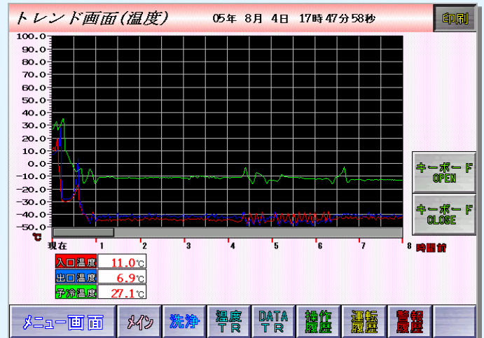
温度トレンド画面
